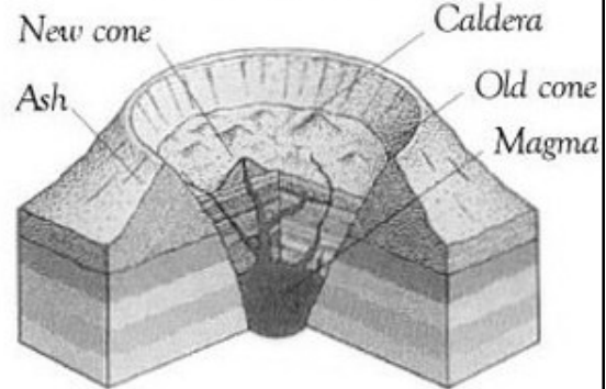
Caldera volcano
